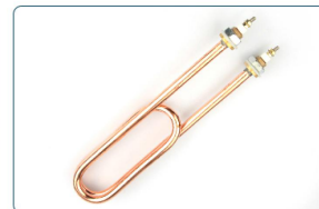
best-f12
